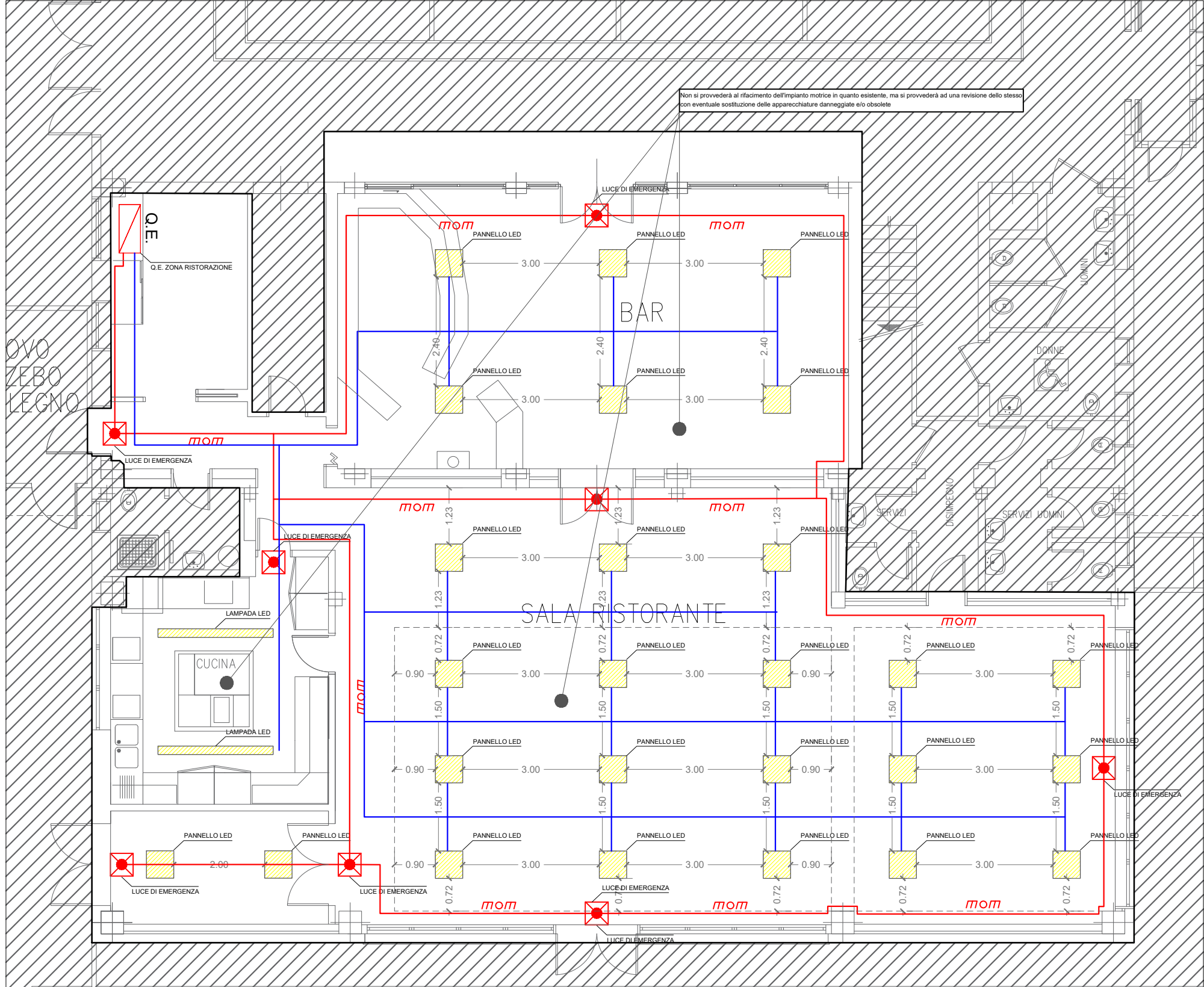
PIANTA SCALA 1:100
