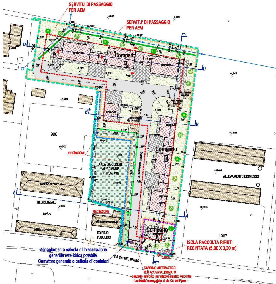
Estratto Tav 2 Planivolumetrico
